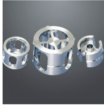
JAUHAS DE VÁLVULAS DE SUCCIÓN Y DESCARGA
